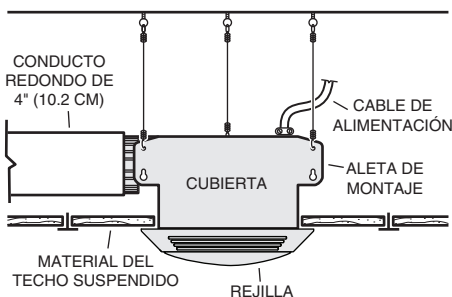
TECHOS SUSPENDIDOS Cubierta montada con cables. Montaje de tres puntos.
